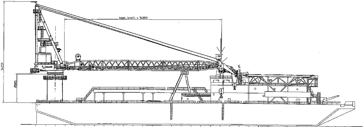
ВИД СБОКУ
