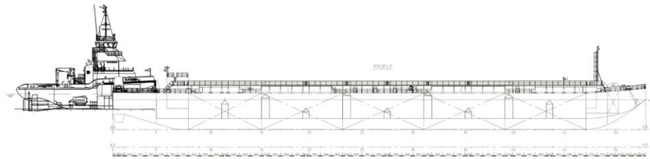
ВИД СБОКУ
