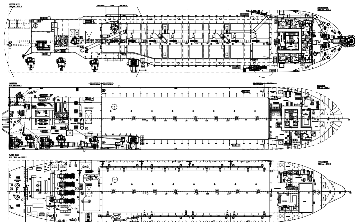
ВИД СВЕРХУ
