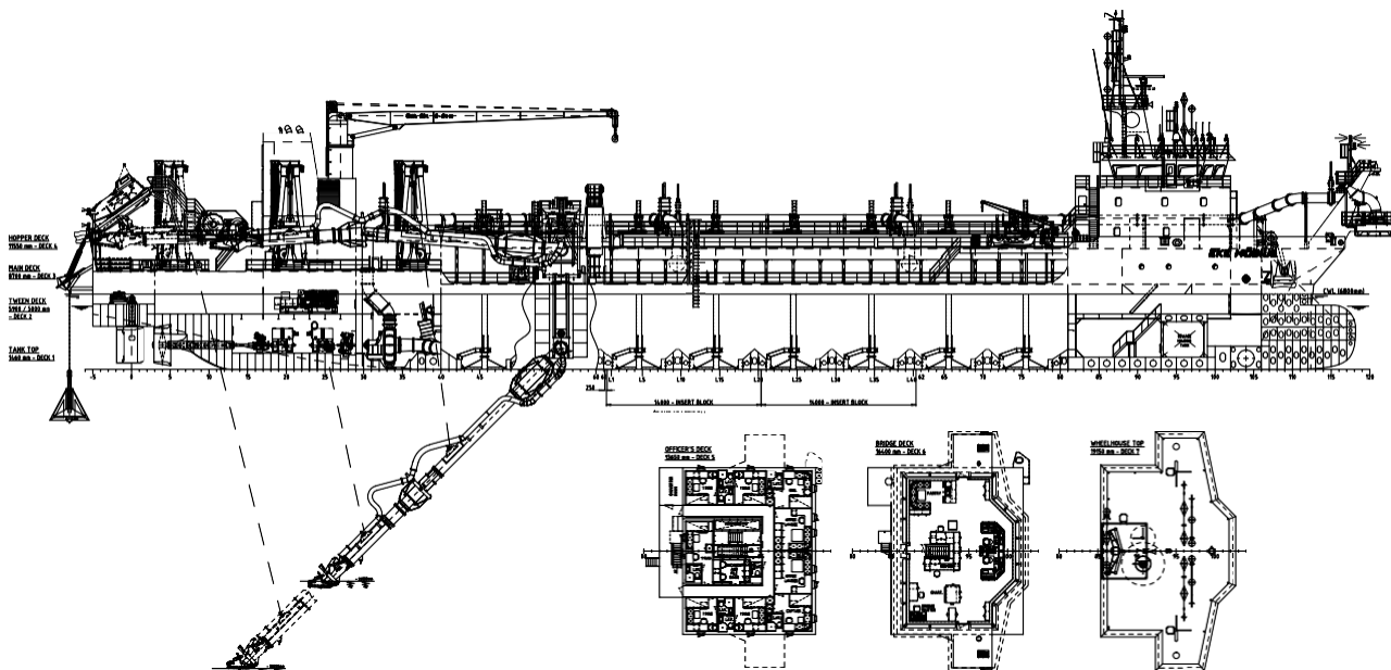
ВИД СБОКУ
