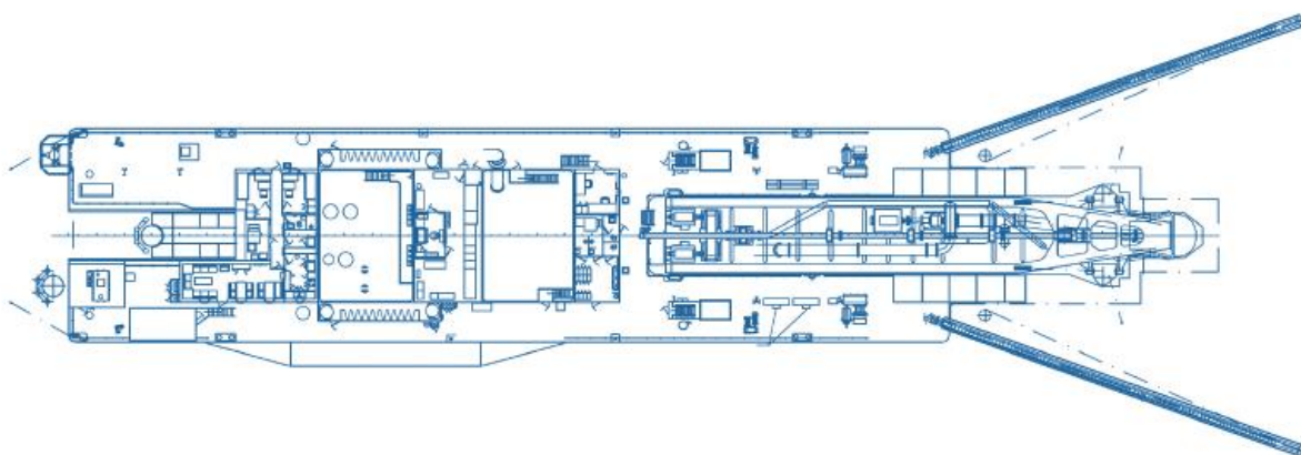
ПАЛУБА. ВИД СВЕРХУ
