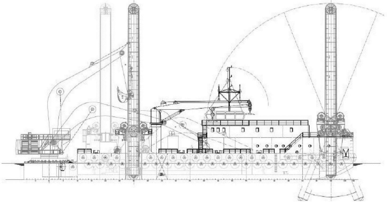
ВИД СБОКУ
