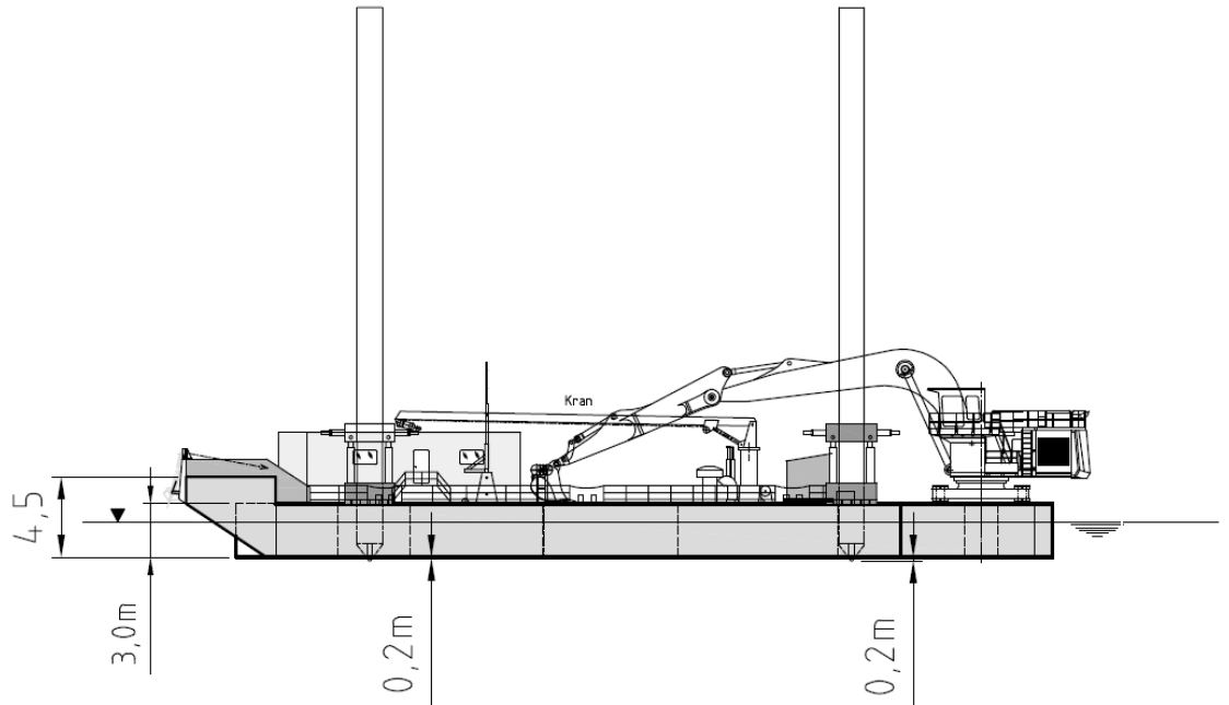
Вид сбоку
