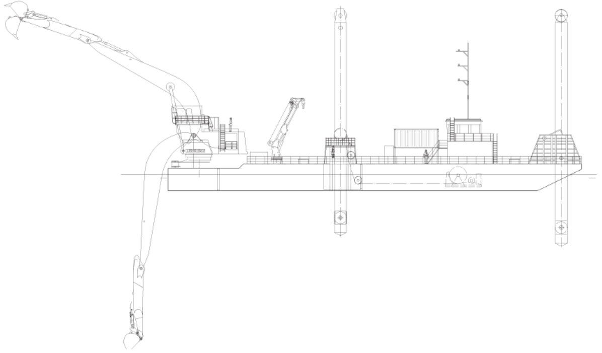
ВИД СБОКУ
